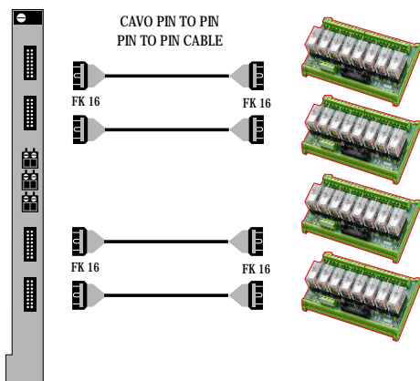
FRONTALE SIEMENS - FRONT COVER 6ES7-921-4AA-0AA0 6ES7-921-4AB-0AA0
